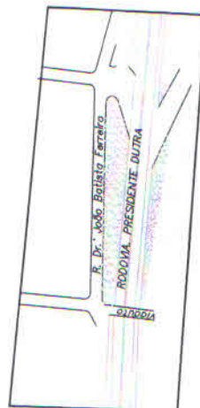
PLANTA DE LOÇÃO S/ ESC
